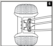
Remontez la biellette de direction, les joints à rotule, l'étrier de frein, l'écrou à essieu, le pneu et la roue.
