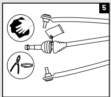
Videz le sachet de graisse dans le joint homocinétique/soufflet, nettoyez les points d'étanchéité et installez les colliers de serrage.
