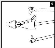
Étalez le lubrifiant à base de silicone sur toute la surface de l'outil conique. Glissez le soufflet sur l'outil conique en commençant par le côté plus large. Consultez les instructions pour le soufflet extérieur sur l'emballage.
